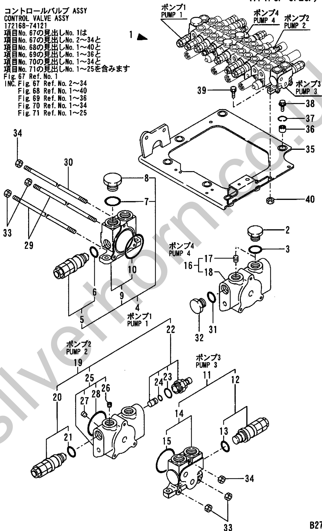
Fig. 67 67 コントロールバルブ(Pポート & バルブ台:PT0仕様) CONTROL VALVE(P PORT & VALVE STAND :P. T. O. SPEC.)
