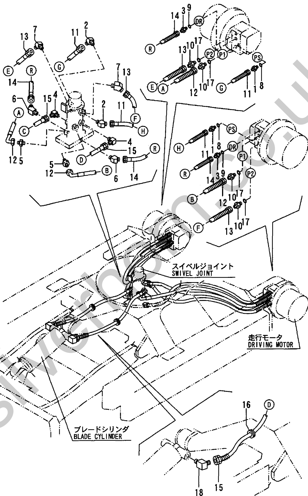
Fig. 85 油圧配管(トラックフレーム) HYD. OIL PIPING (TRACK FRAME)
