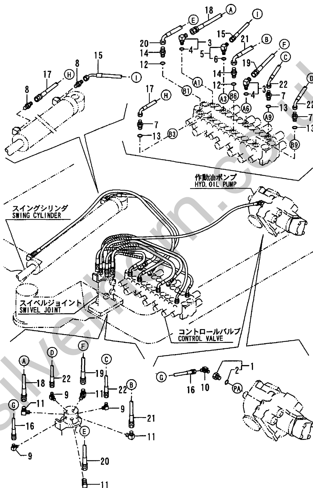
Fig. 81 油圧配管(バルブ～スイベル, スイグ) HYD. OIL PIPING (VALVE~SWIVEL, SWING)
