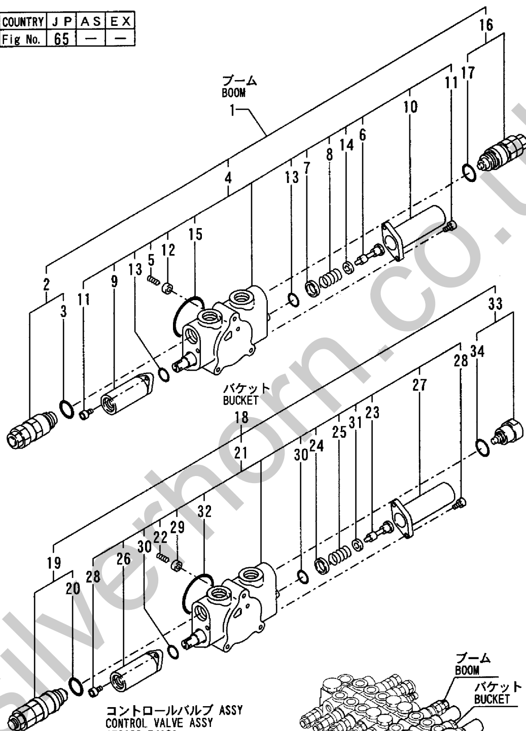
Fig. 65 コントロールバルブ(ブーム & バケット:標準仕様) CONTROL VALVE (BOOM & BUCKET: STANDARD SPEC.)
