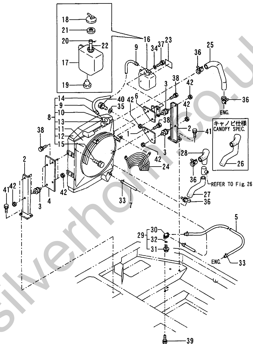
Fig. 17 ラジエータ & マウント RADIATOR & MOUNT
