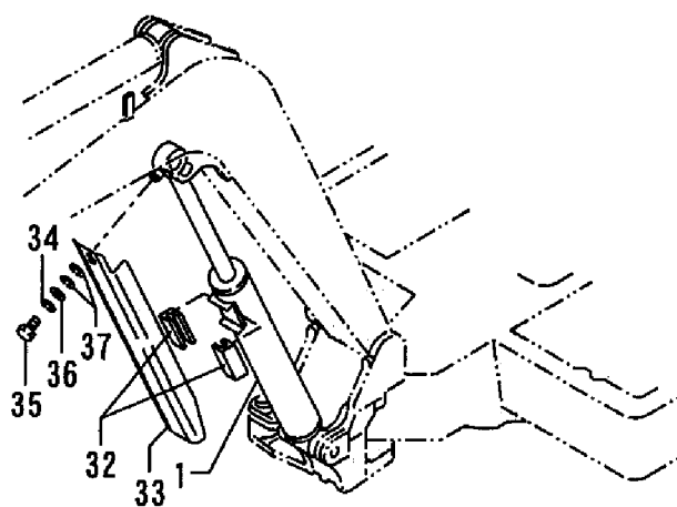
Fig. 54 ブームシリンダ(キャパ°) BOOM CYLINDER (CANOPY)
