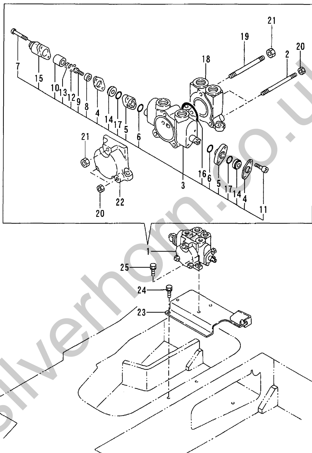
Fig. 77 P.T.O.バルブ(合流) P.T.O. VALVE (CONFLUENCE)
