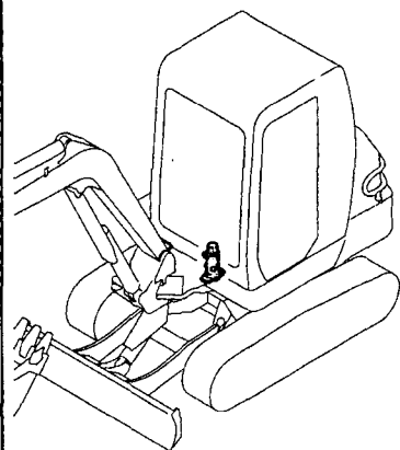
Fig. 62 コントロールバルブ (Pポート & バルブ台:標準仕様) CONTROL VALVE (P PORT & VALVE STAND: STANDARD)
