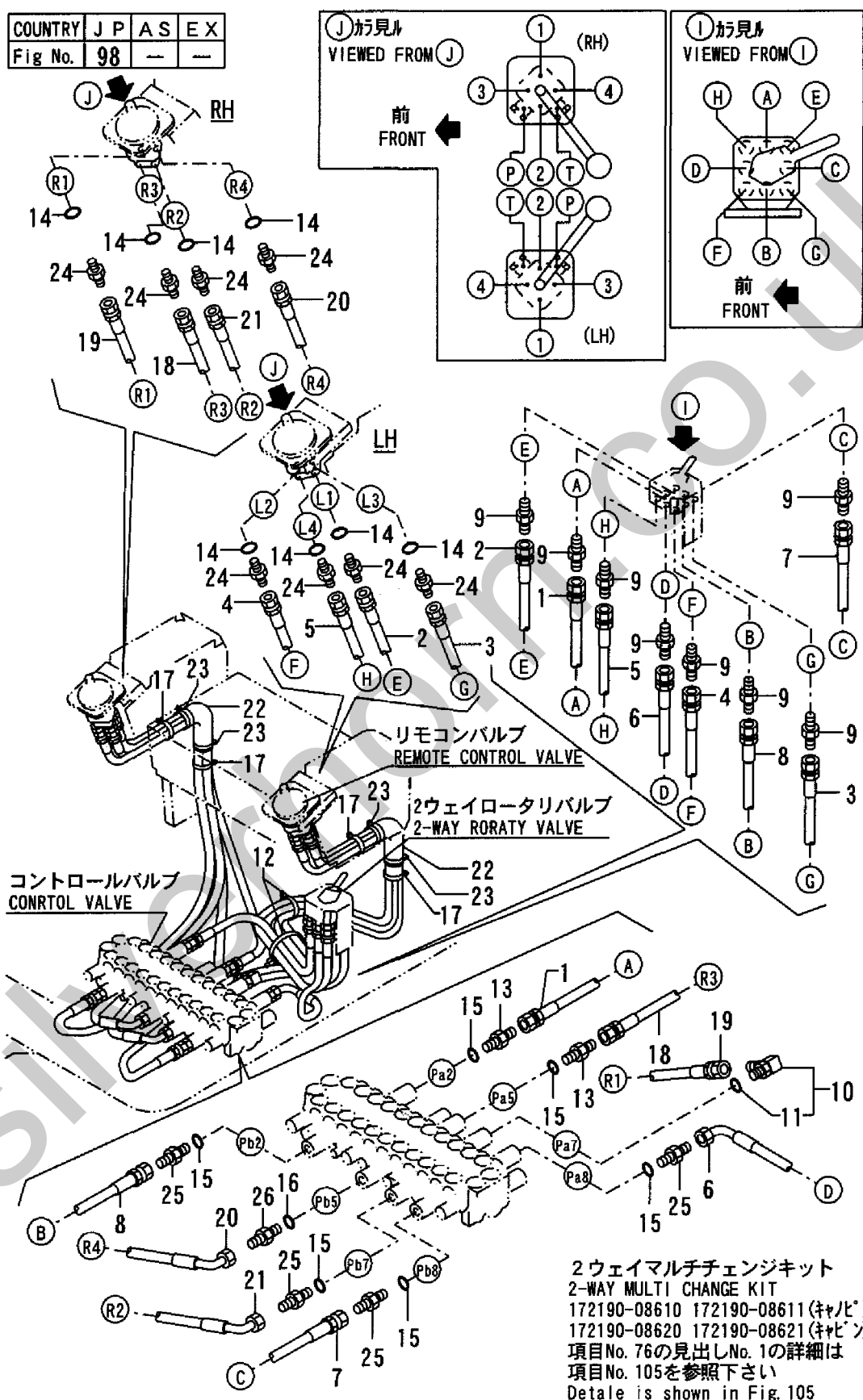
Fig. 98 コントロール配管(マルチチェンジ:2ウェイ, サイドレバー) CONTROL PIPING(MULTI CHANGE:2-WAY, SIDE LEVER)
