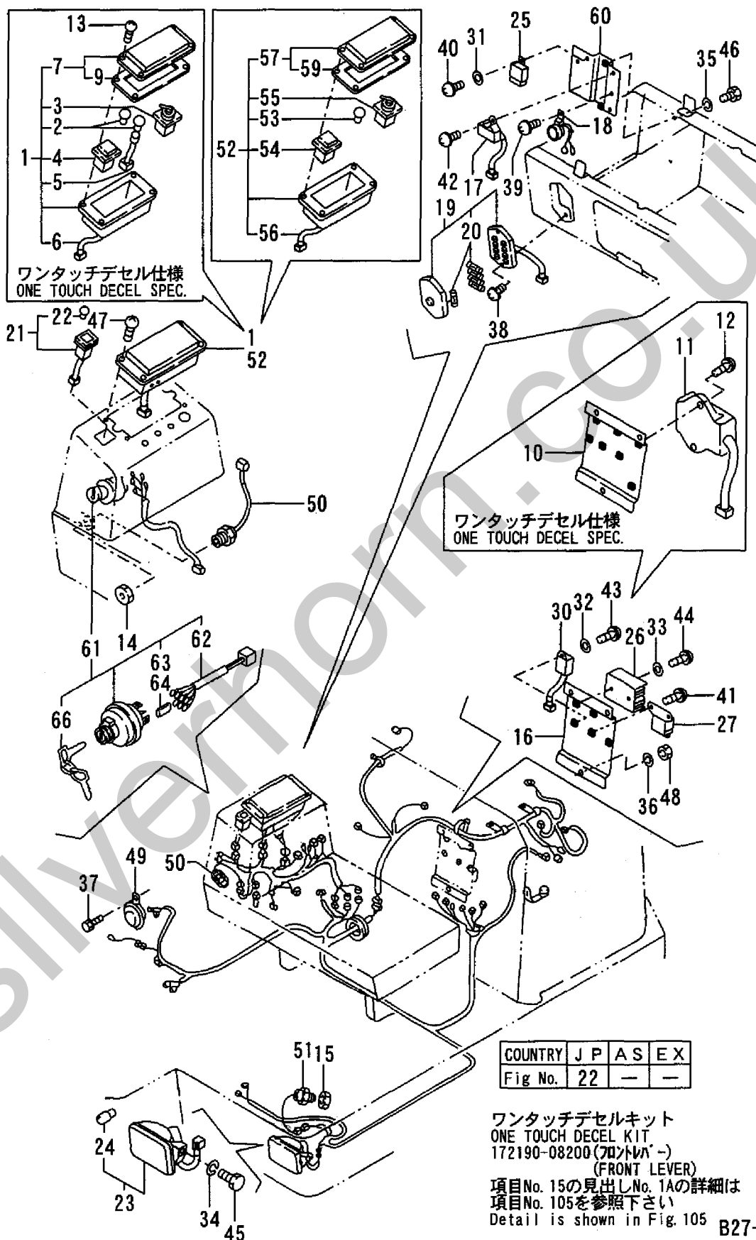
Fig. 22 電装品 (機器: フロントレバー) ELECTRIC PART (EQUIPMENT: FRONT LEVER)
