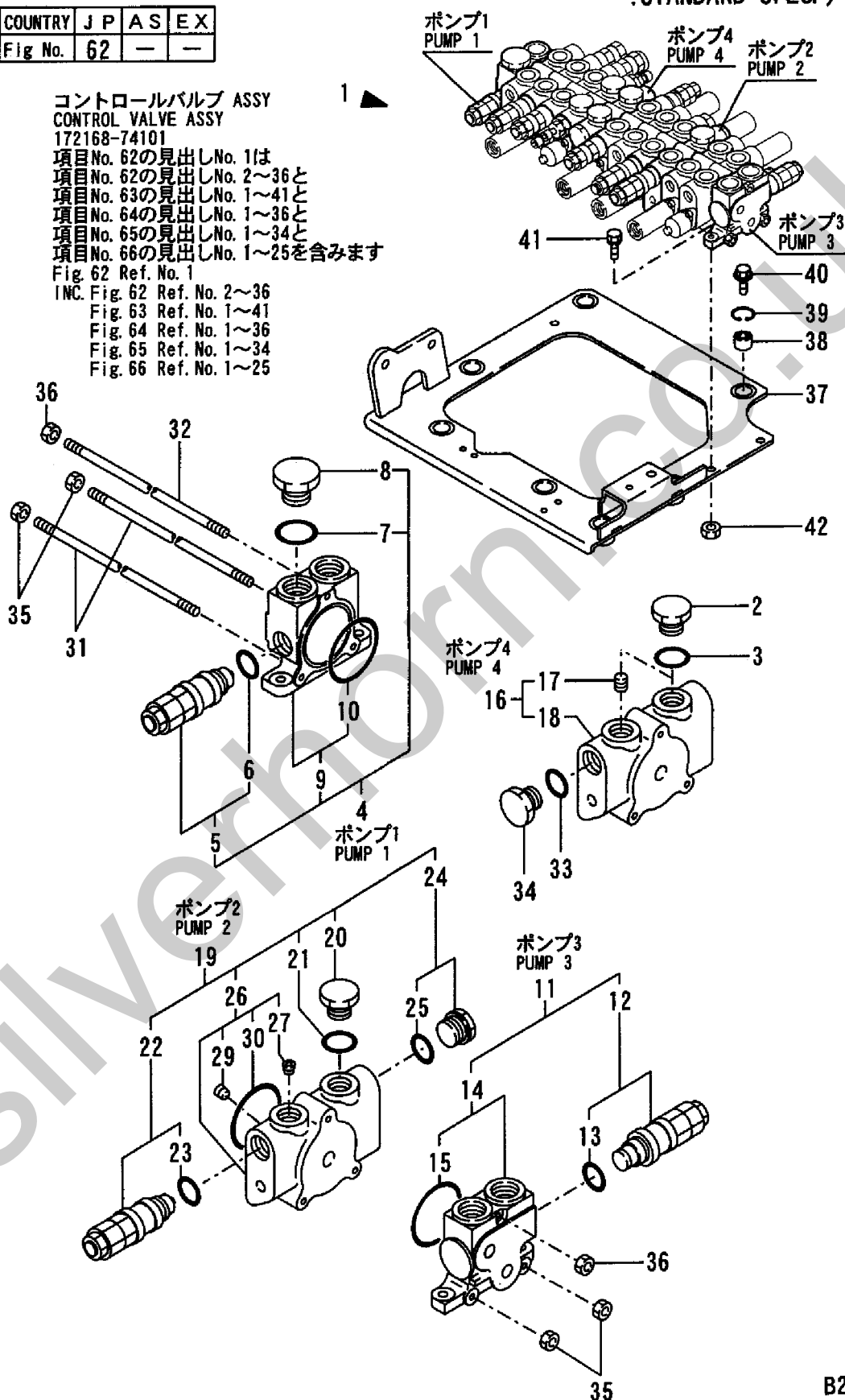
Fig. 62 62 コントロールバルブ (Pポート & バルブ台:標準仕様) CONTROL VALVE (P PORT & VALVE STAND :STANDARD SPEC.)
