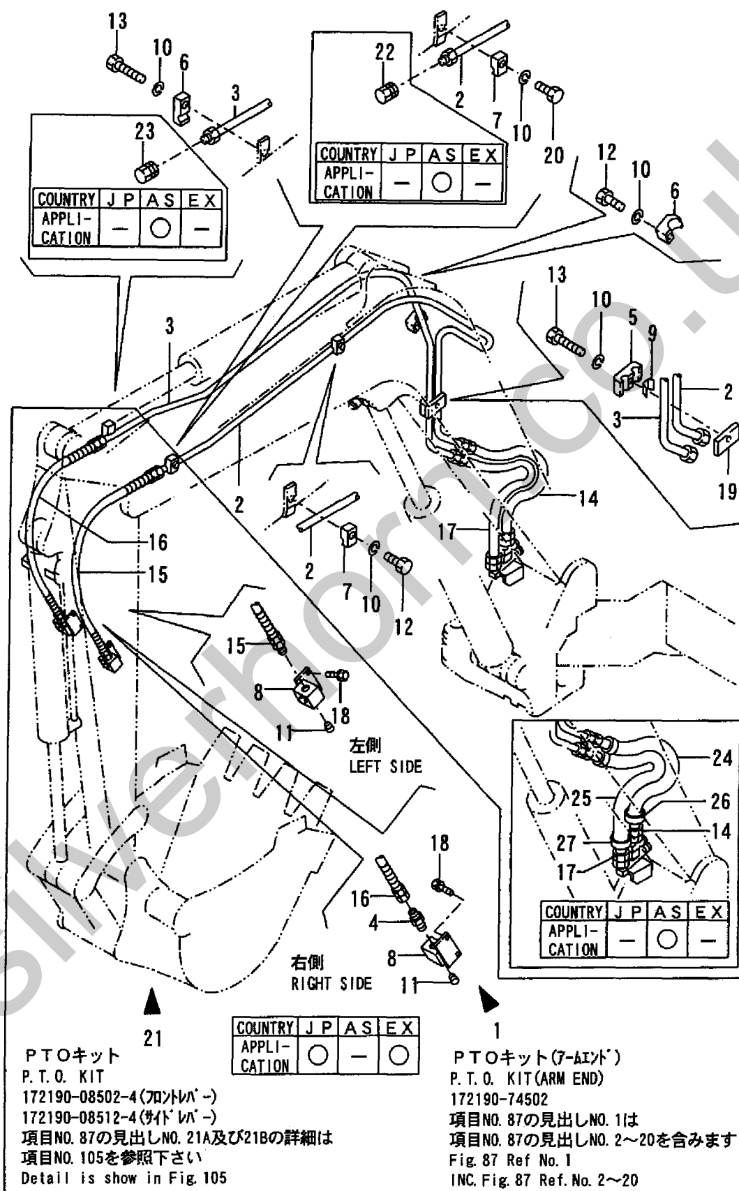
Fig. 87 油圧配管 (PTO アーム) HYD. OIL PIPING (P. T. O. ARM END)
