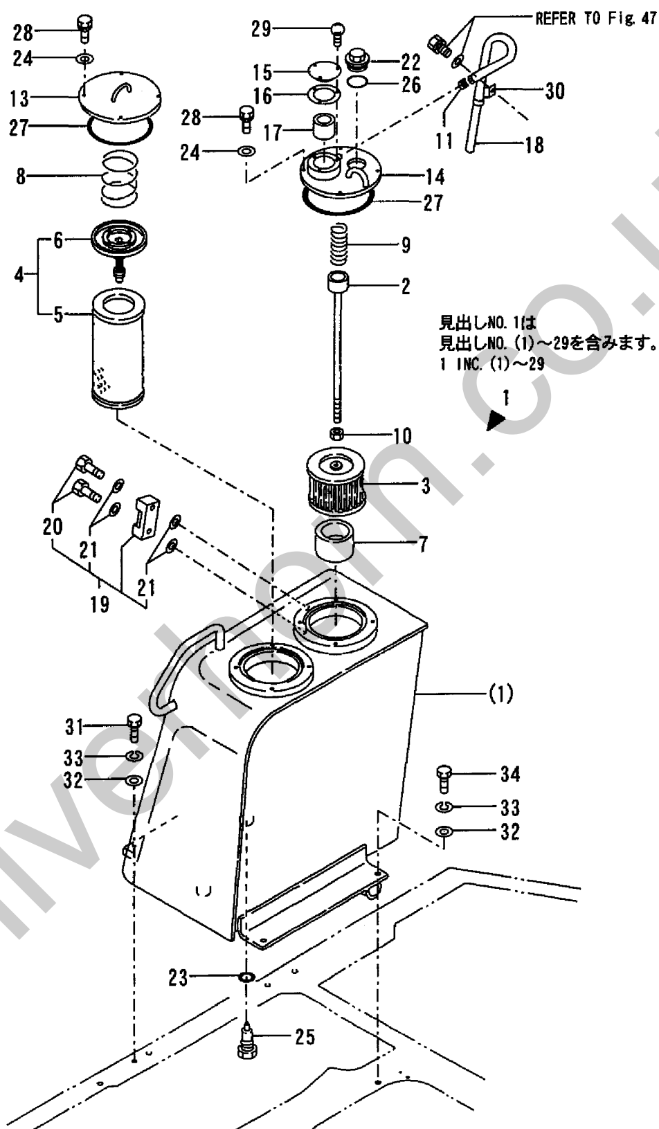
Fig. 78 作業油タンク HYD. OIL TANK
